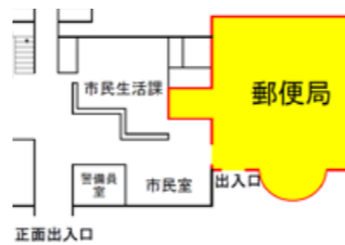
▲輝北総合支所1階配置図
