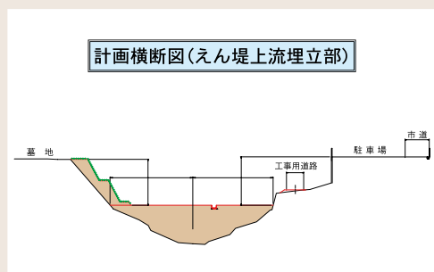
計画横断面図
