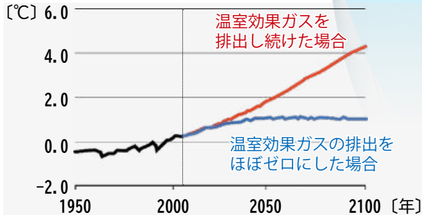
▼世界平均地上気温のシミュレーション
