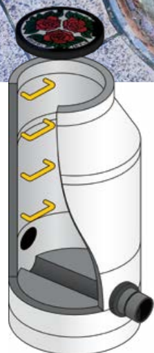
▲下水道マンホールの構造
