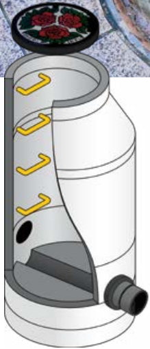
▲下水道マンホールの構造
